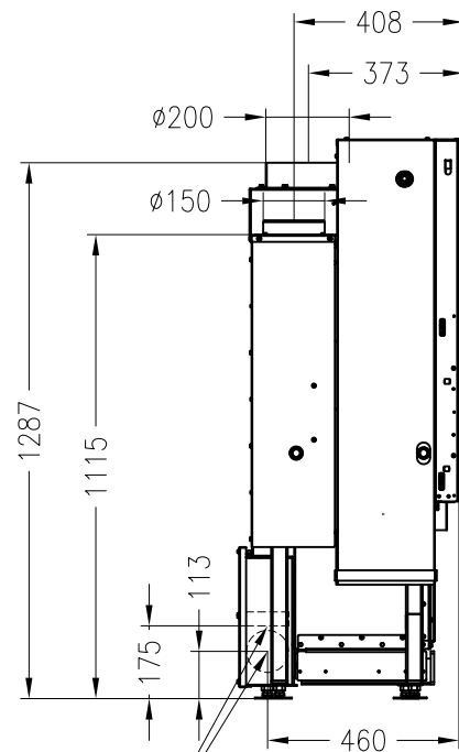
Seitenansicht M~1:20
