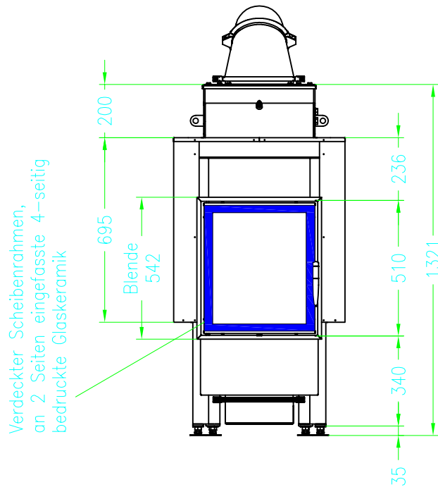
Vorderansicht M~1:20
