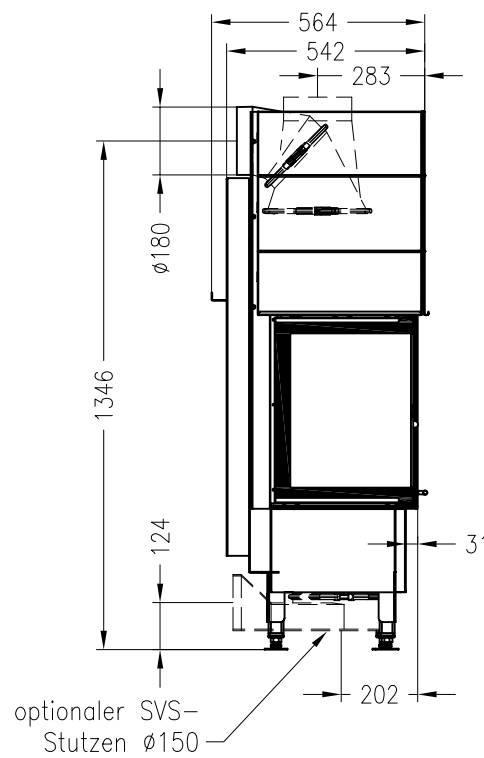
Seitenansicht M~1:20
